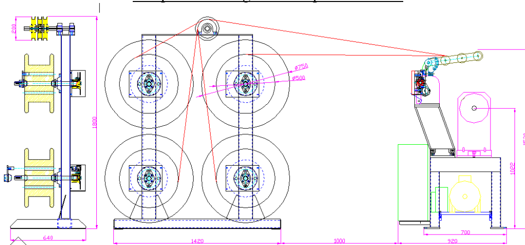
Beispielzeichnung einer 4-Spulen Version
